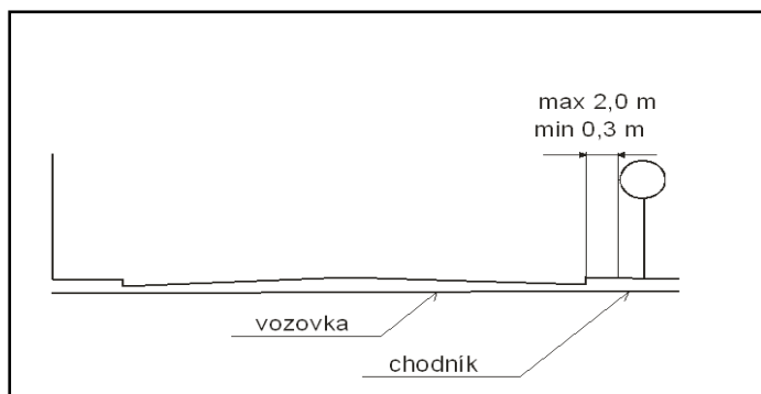
Obr. č.1. Umiestnenie dopravného značenia
